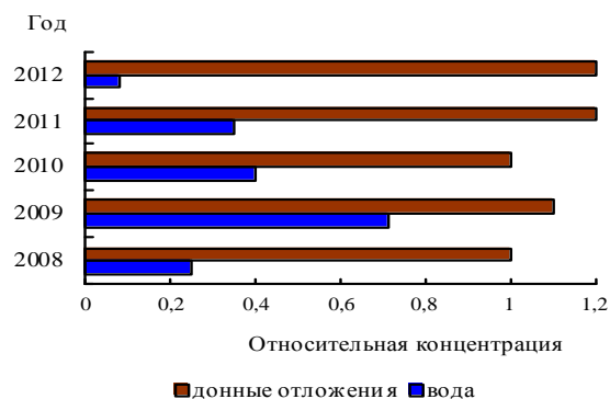
Относительная концентрация тяжелых металлов в воде (кратность ПДК) и донных отложениях (кратность СХК) Нижнего Дона
